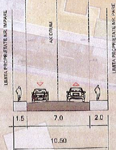
Profil Existent și Menținut Strada Logofătul Dan Scara 1:250
