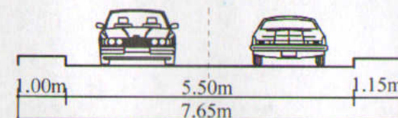
Profil existent (D-D')
