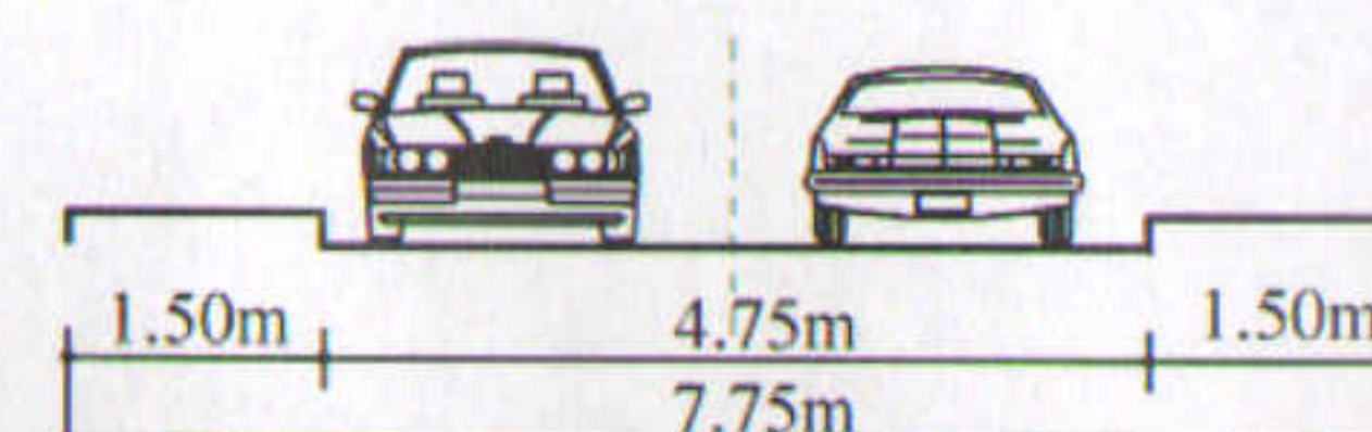
Profil existent (A-A') Aleea Magura Vulturului (Intr. Melitei)
