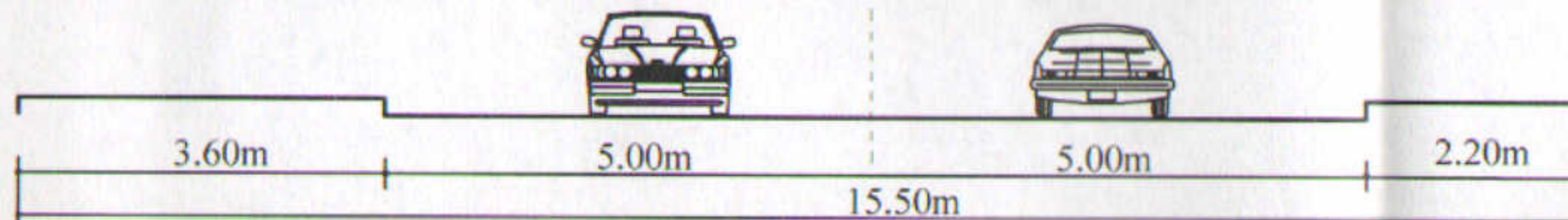
Profil existent (C-C') str. Avrig
