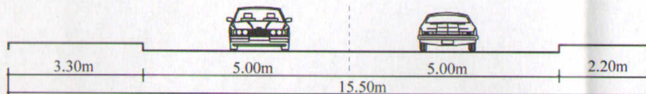
Profil existent (B-B') str. Avrig
