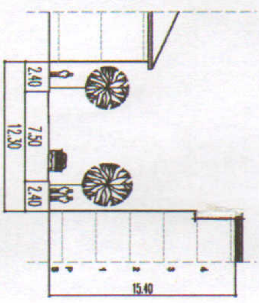
STRADA POPA NAN PROFIL TRANSVERSAL
