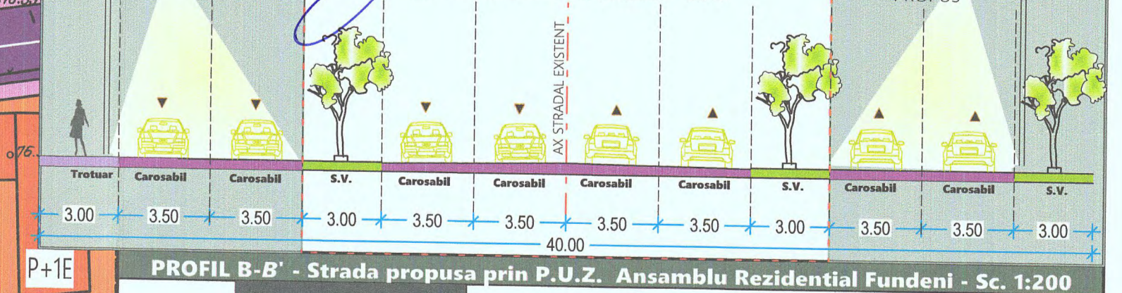
PROFIL B-B' - Strada propusa prin P.U.Z. Ansamblu Rezidential Fundeni - Sc. 1:200
