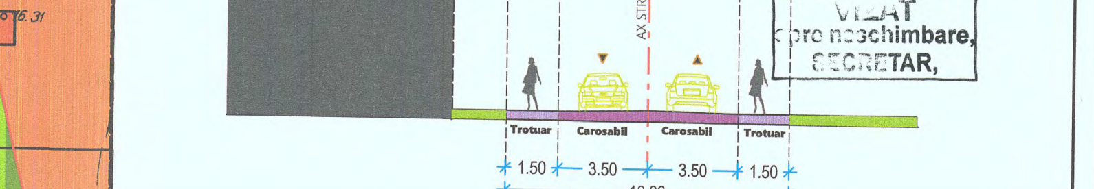
PROFIL B-B' - Strada propusa prin P.U.Z. Ansamblu Rezidential Fundeni - Sc. 1:200
