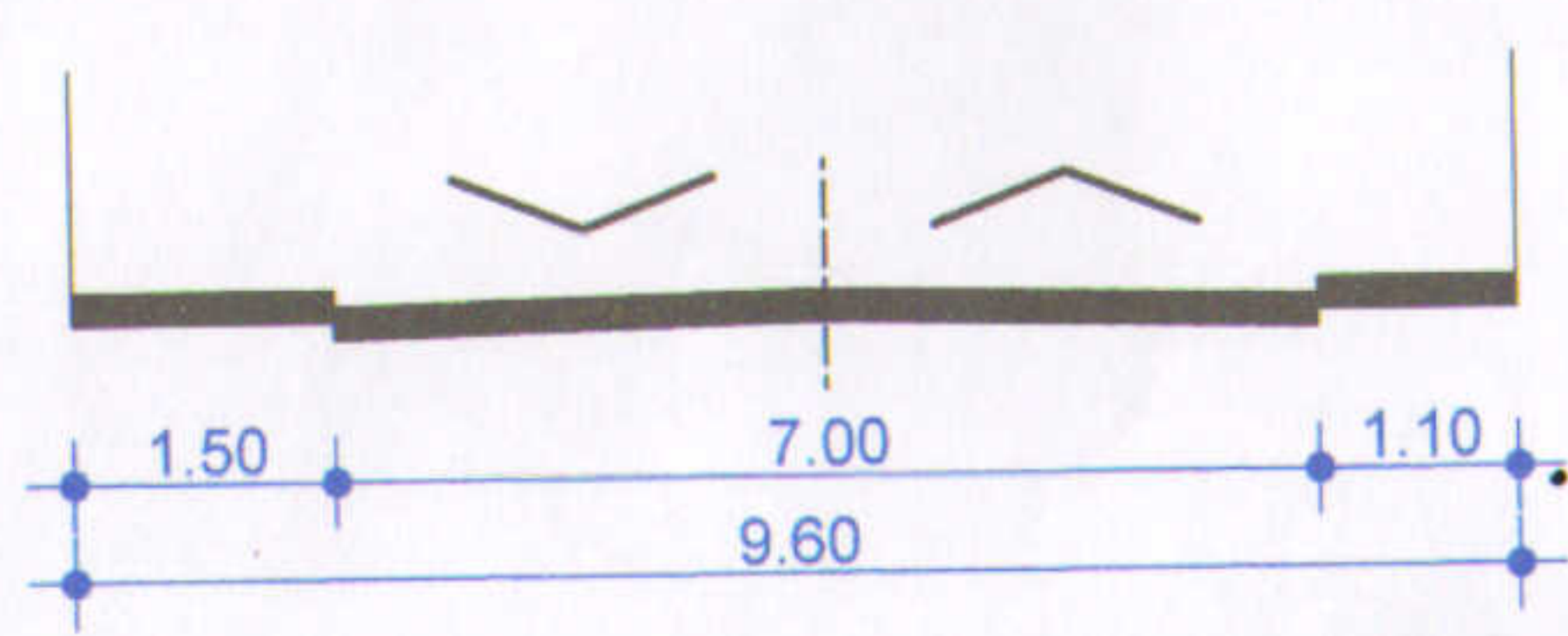
PROFIL STRADAL EXISTENT - Str. Teofil (sectiunea A-A)
