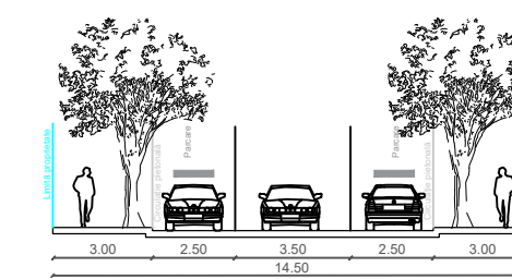
Secțiune strada Prof. Ion Maiorescu A - A'
