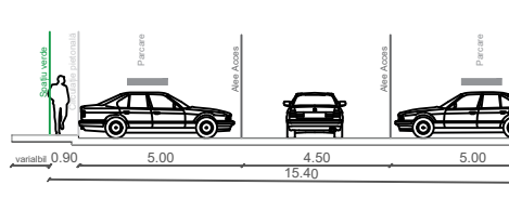
Secțiune stradă acces - Profil transversal B - B'
