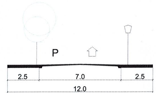
STRADA PARGARILOR Profil existent si mentinut
